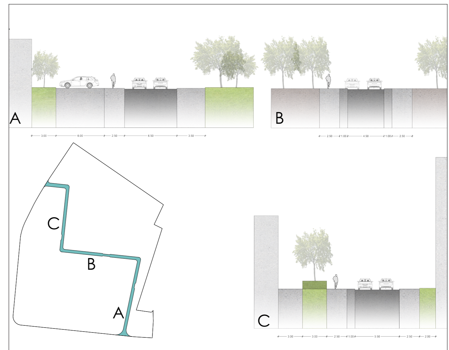
Straßenschnitt
