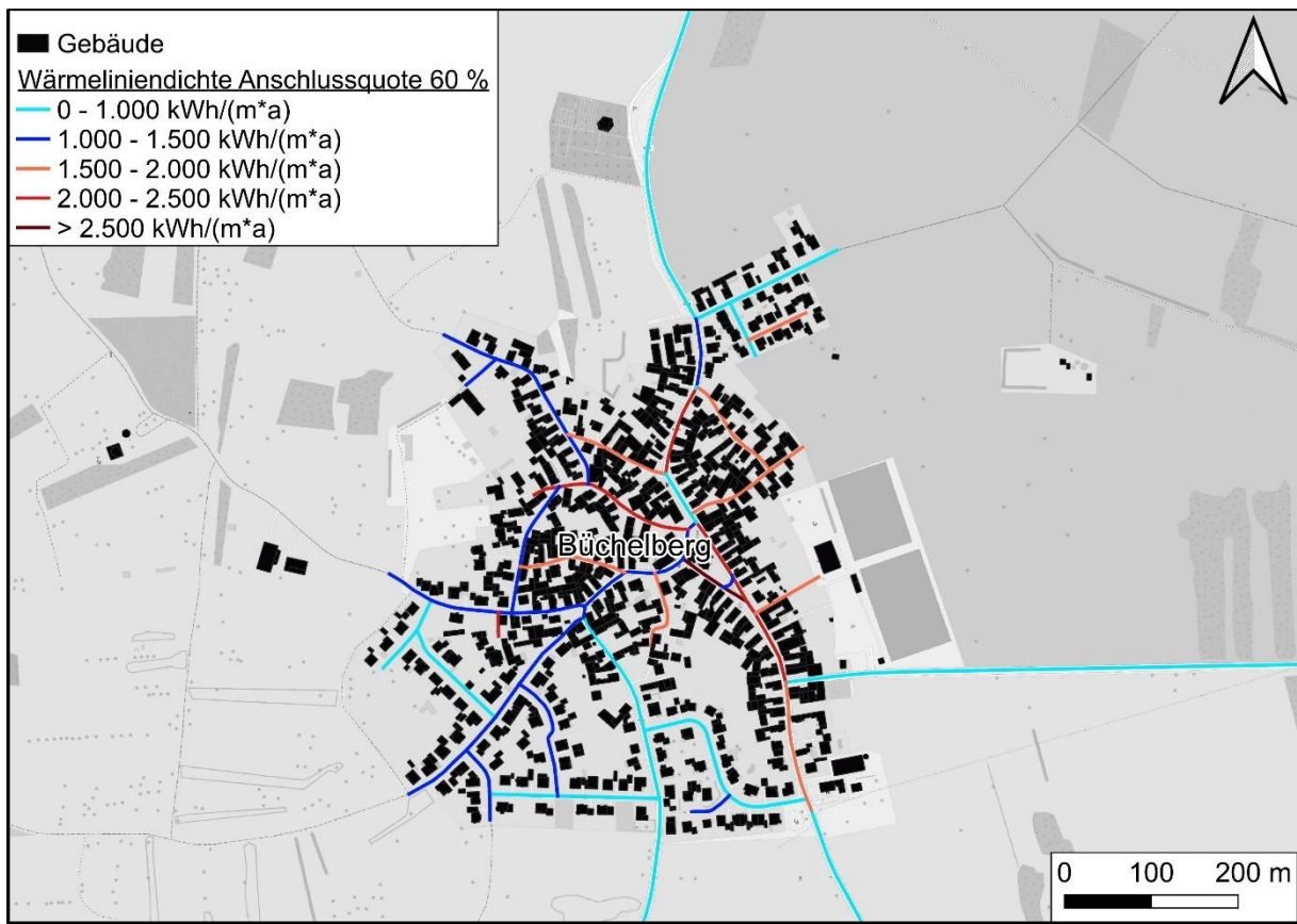
Abbildung 6-10: Wärmelinien dichten im Ortsbezirk Büchelberg
