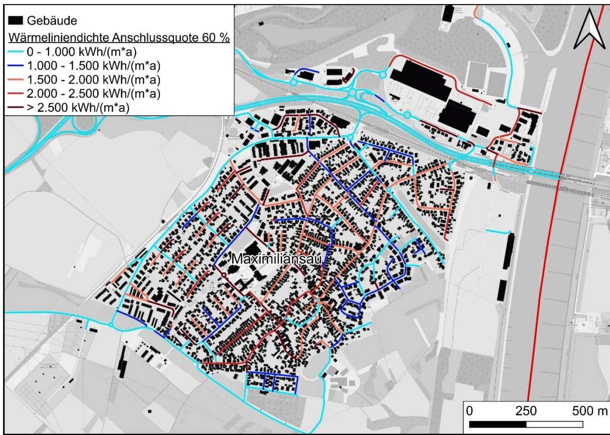
Abbildung 6-6: Wärmelinien dichten im Ortsbezirk Maximiliansau
