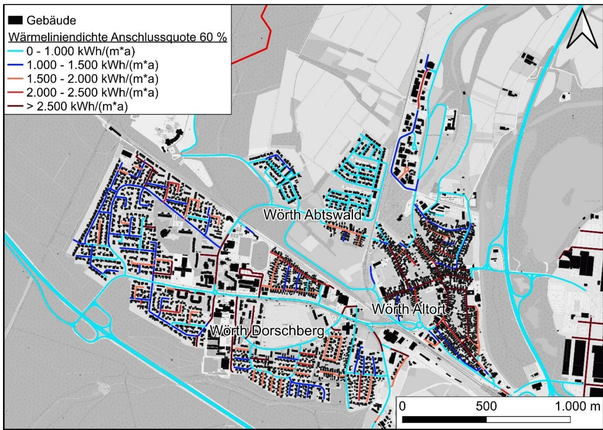
Abbildung 6-4: Wärmelinien dichten in den Gebieten Dorschberg, Altort und Abtswald
