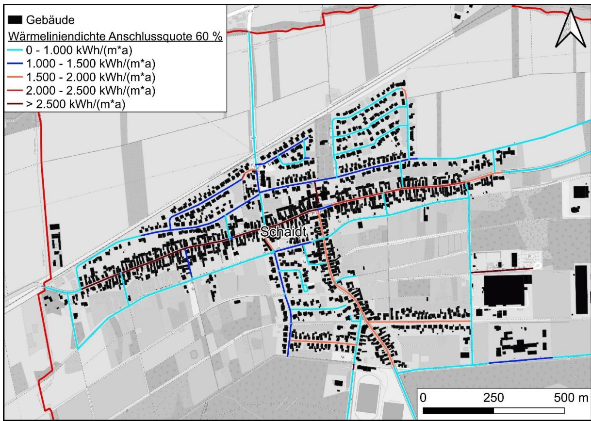
Abbildung 6-8: Wärmelinien dichten im Ortsbezirk Schaidt
