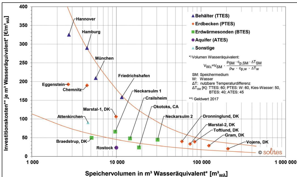
Abbildung 5-26: Kosten von verschiedenen Saisonspeichervarianten pro m 3 .
