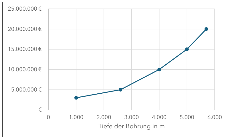
Abbildung 5-22: Kostenfunktion der Bohrkosten für eine Tiefengeothermieanlage. Datenquelle: AFGW Praxisleitfaden Tiefengeothermie
